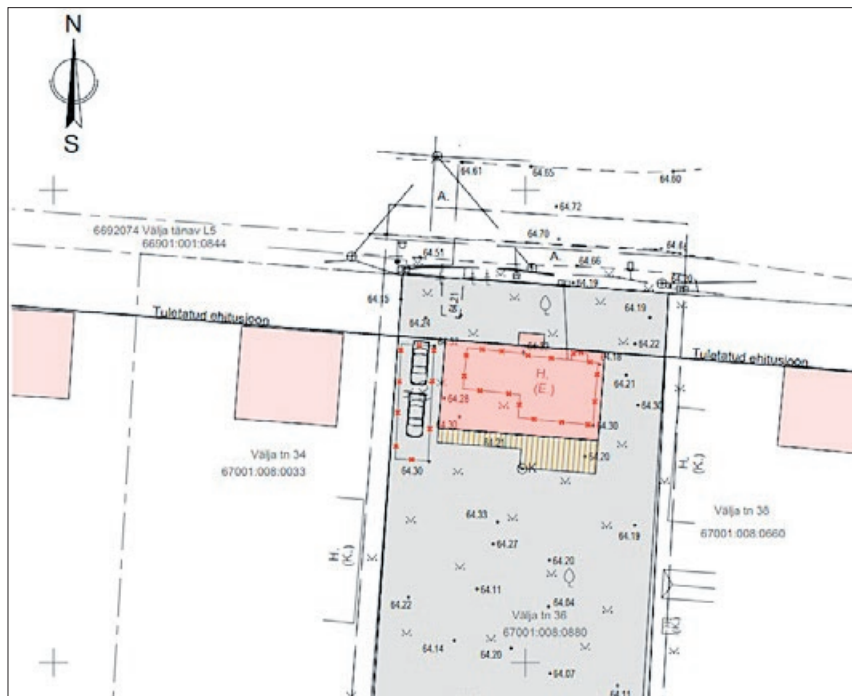
Välja tn 36 asendiplaani eskiis (autor arhitekt Erko Leo).
