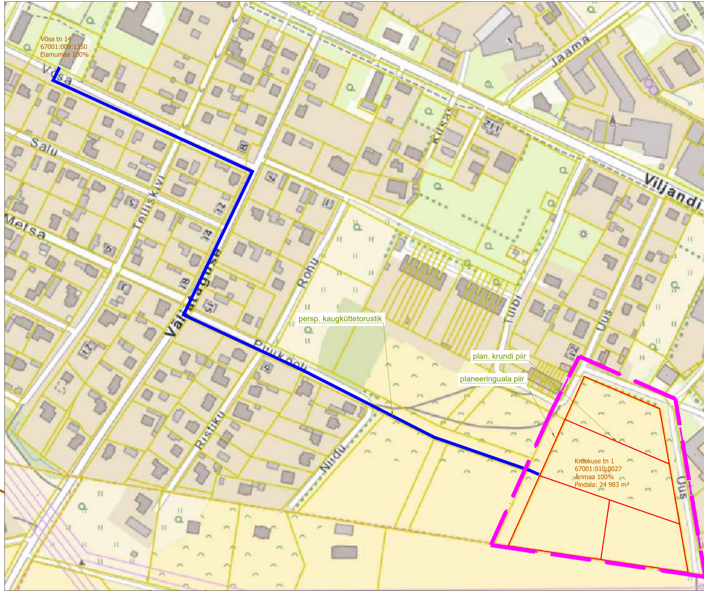
PERSPEKTIVSE KAUGKÜTTETORUSTIKU SKHEEM
