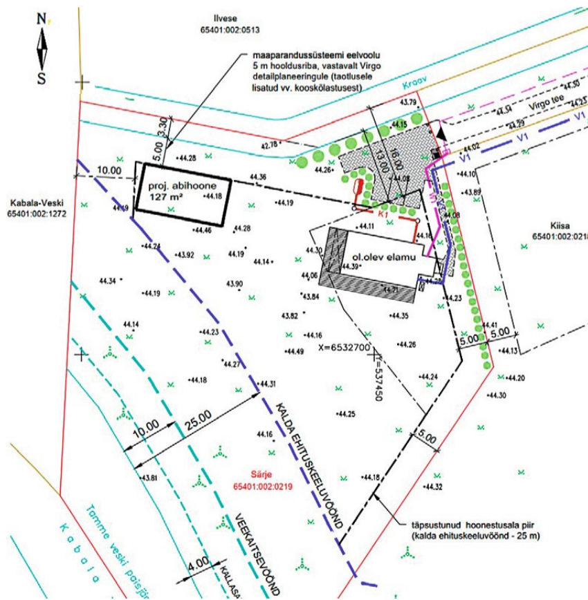
Särje maaüksuse kavandatud asendiplaneiline lahendus (autor arhitekt Tõnis Sirp, osahing TS-Projektbüroo töö).
